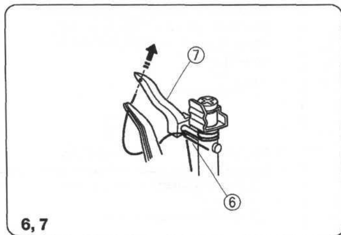
(6) Нитенаправитель верхнего петлителя (7) Верхний петлитель
