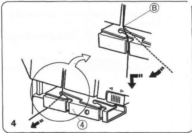
(4) Нитенаправитель петлителя
