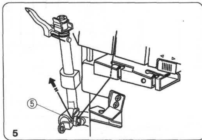
(5) Натяжитель нити петлителя (верхний)
